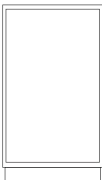
CAISSON BAS SIMPLE sans porte L.500 x P.550 x H.880 mm RÉF. : 372.5701
