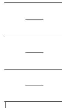
CAISSON BAS SIMPLE 3 tiroirs L.500 x P.550 x H.880 mm RÉF. : 372.5703
