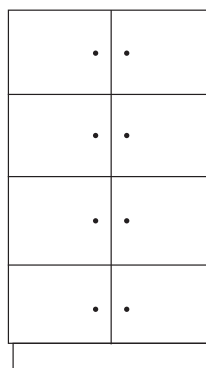
CAISSON BAS 8 CASIERS L.500 x P.320 x H.880 mm Avec portes RÉF. : 372.57011 Sans porte RÉF. : 372.57010
